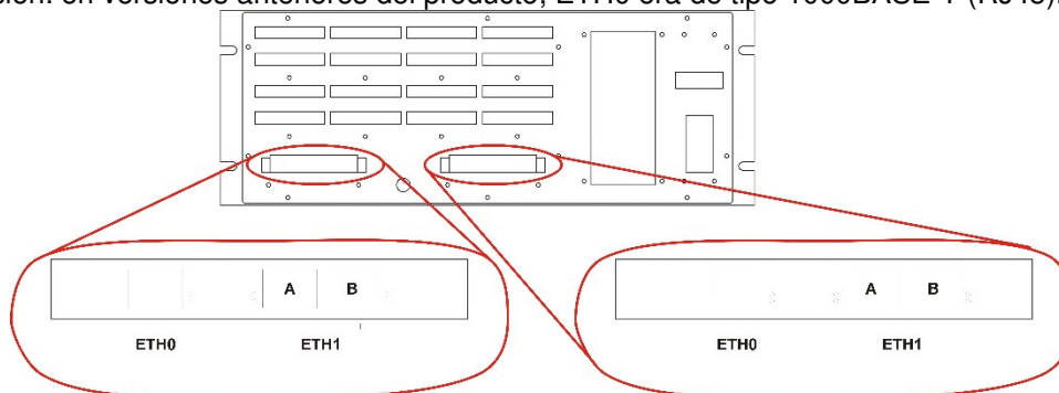
Figura 3-18 : Módulos SV - Disposición
