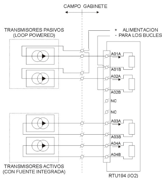
Figura 3-12 : Módulos IO2 - EA - Ejemplos de Conexionado
