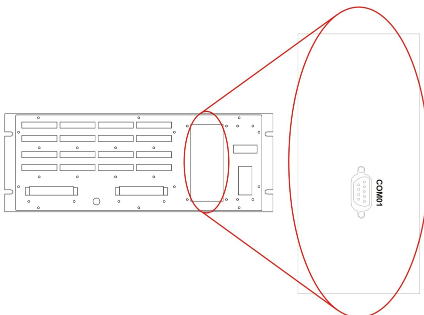
Figura 3-7 : Comunicaciones CNC
