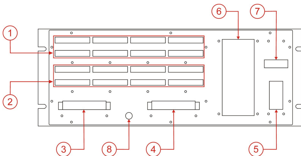
Figura 3-2 : Vista posterior de RTU194
