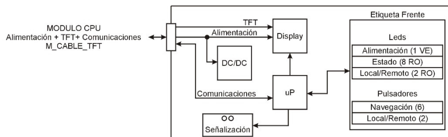
Figura 4-4 : Arquitectura Módulo DISPLAY
